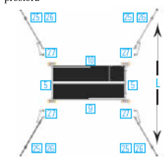
od typu lešení 2126-2151 odstup L_{min}=3,20 m
