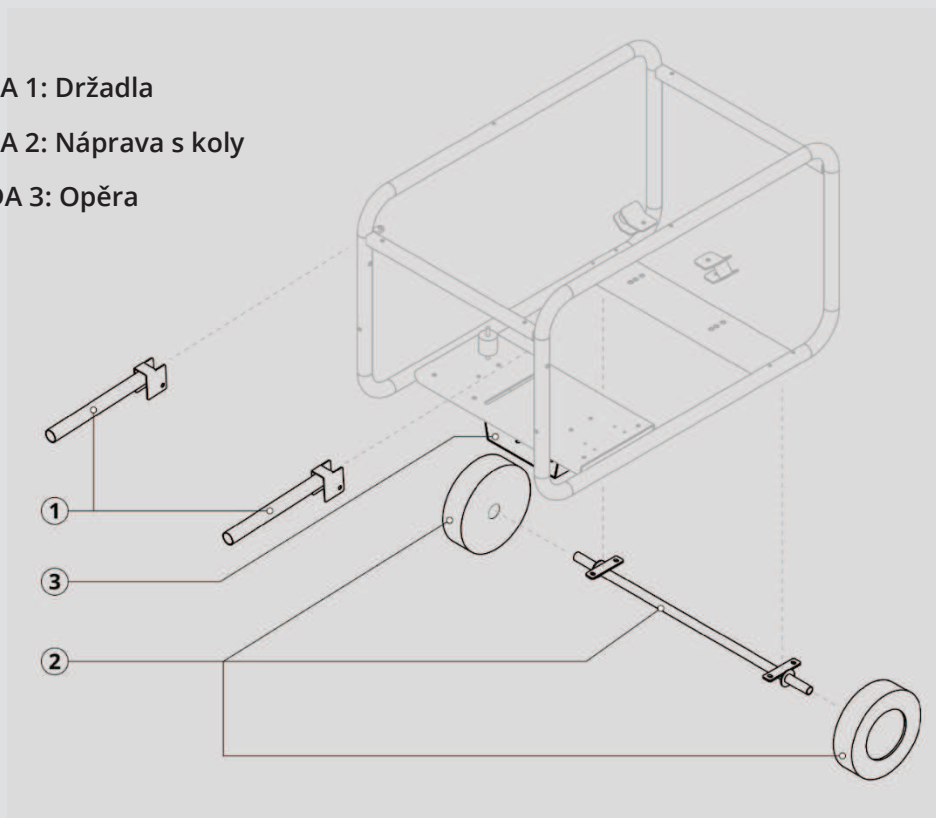
Obrázek 18: Součásti přepravního podvozku Dagartech
