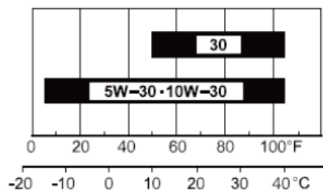
Obrázek 8: Graf použitelnosti viskozitních tříd motorových olejů podle okolní teploty
