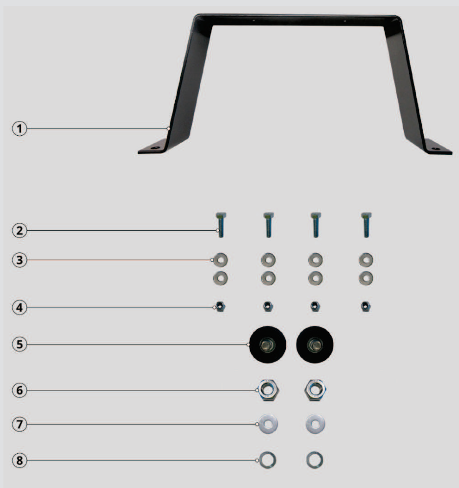
Obrázek 21: Seznam součástí Sada 3: Opěra
