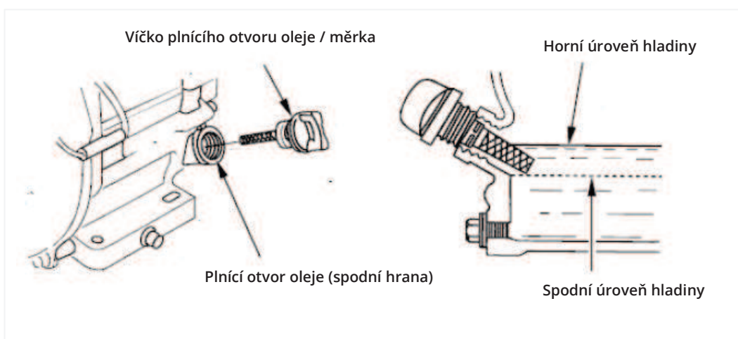
Obrázek 9: Postup kontroly množství oleje
