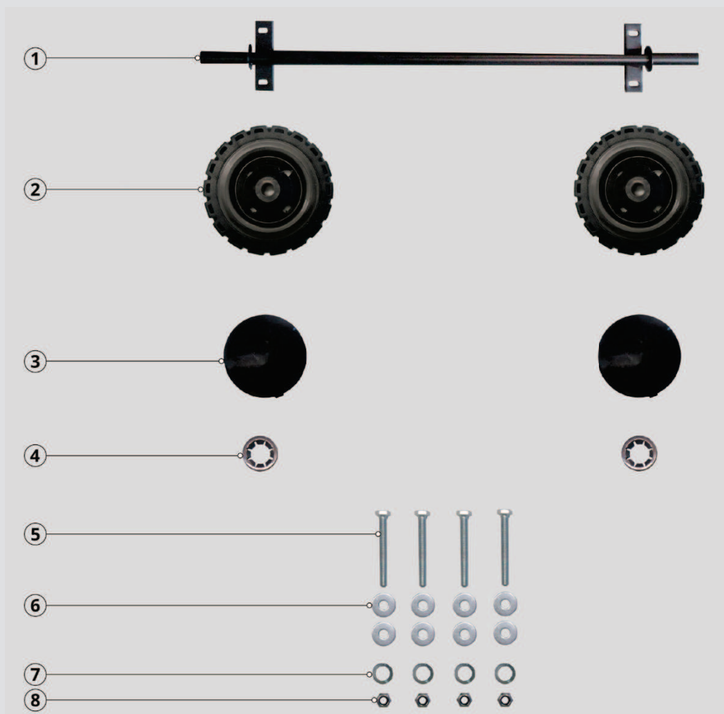
Obrázek 20: Seznam součástí Sady 2: Náprava s koly
