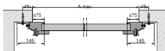
Montáž s volitelnou speciální kotvou na boční stěně garáže.
