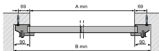
Montáž na úhlovou kotvu
