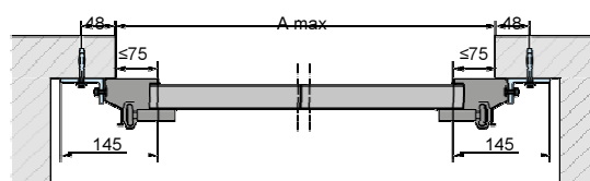
Montáž s volitelnou speciální kotvou na boční stěně garáže.
