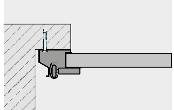
Standardní montáž skrz zárubeň
