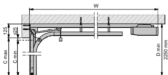
Svislý řez
