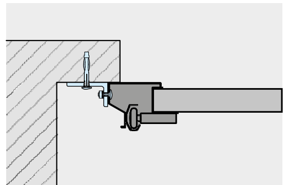
Montáž zárubní přesahujících do otvoru. Kotvení pomocí úhelníkové kotvy, která je součástí dodávky. Maximální povolený přesah zárubně = 75 mm viz výkres na poslední straně.
