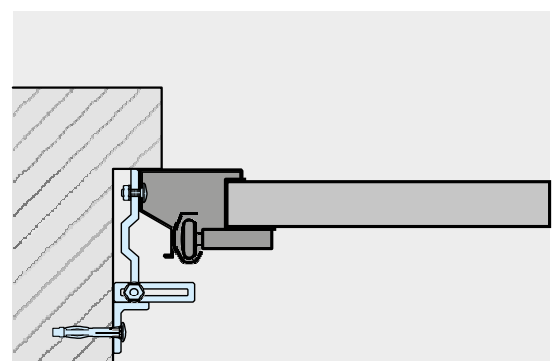
Montáž s volitelnou speciální kotvou na boční stěně garáže. (není součástí dodávky)
