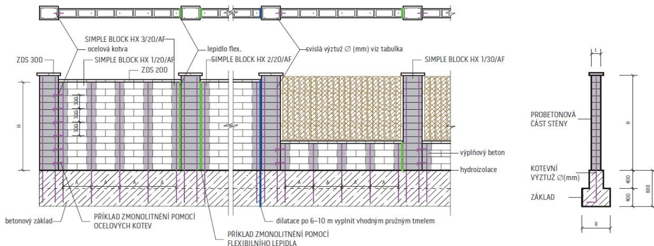
Tabulka: Návrh šířky základu, svislé výztuže a jejich vzdáleností pro stěny zděné systémem SIMPLE BLOCK Schéma probetonování varianta 2
