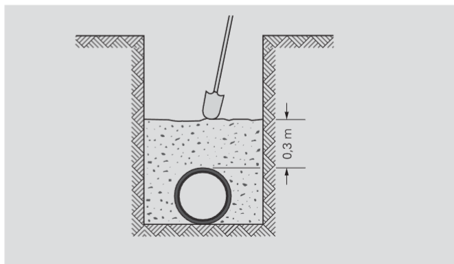
Potrubi do 30 cm nad vrcholem trubky ručně zasypte zhutnitelnou zeminou bez kamení a zhutněte.
