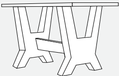
STŮL KOMPLET, DESKA VYMÝVANÁ 160 × 80 × 75
