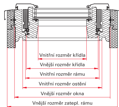
řez B-B
