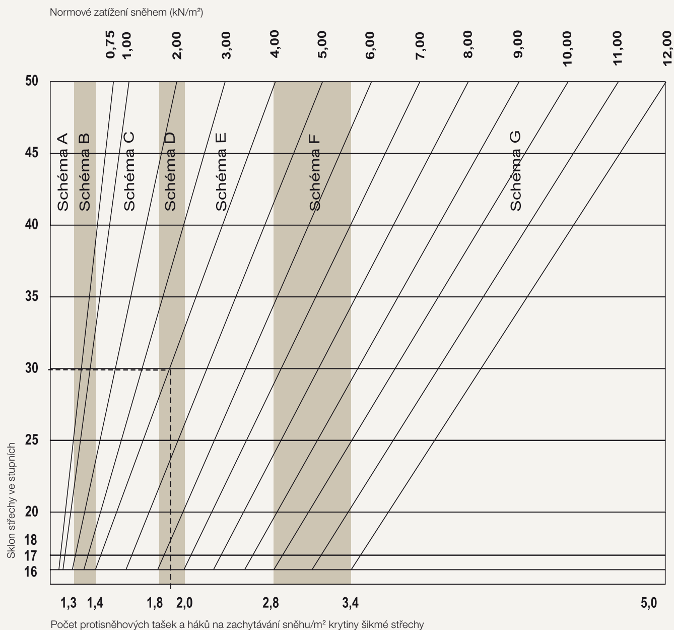
ORIENTAČNÍ VÝPOČET POTŘEBNÉHO MNOŽSTVÍ PROTISNĚHOVÝCH TAŠEK A HÁKŮ V ZÁVISLOSTI NA SKLONU STŘECHY A SNĚHOVÉ OBLASTI
