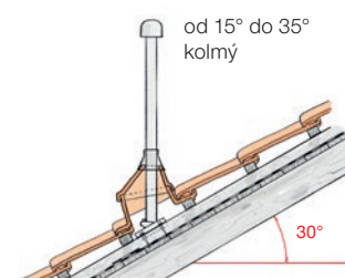
Anténní nástavec s držákem satelitní antény
