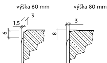
Řez hranou - hladký povrch
